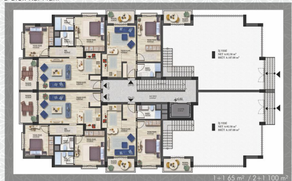
B Blok Kat Planı
