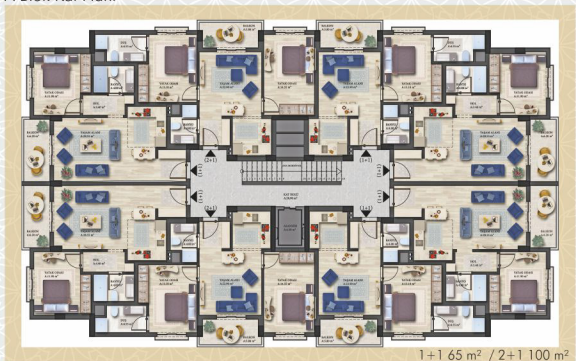
A Blok Kat Planı
